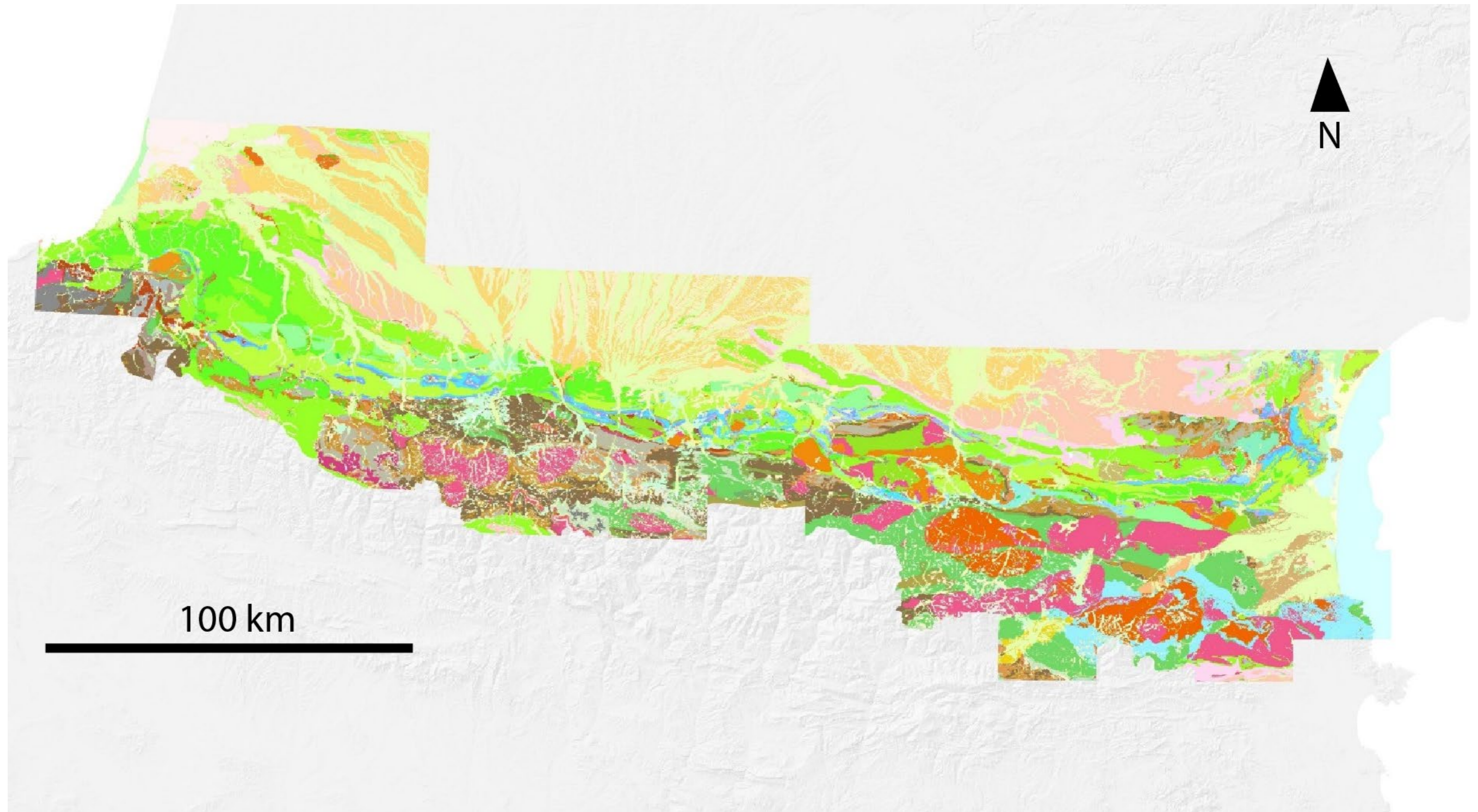
Carte simplifiée des formations géologiques de type "groupes" identifiées dans le cadre du chantier RGF-Pyrénées
