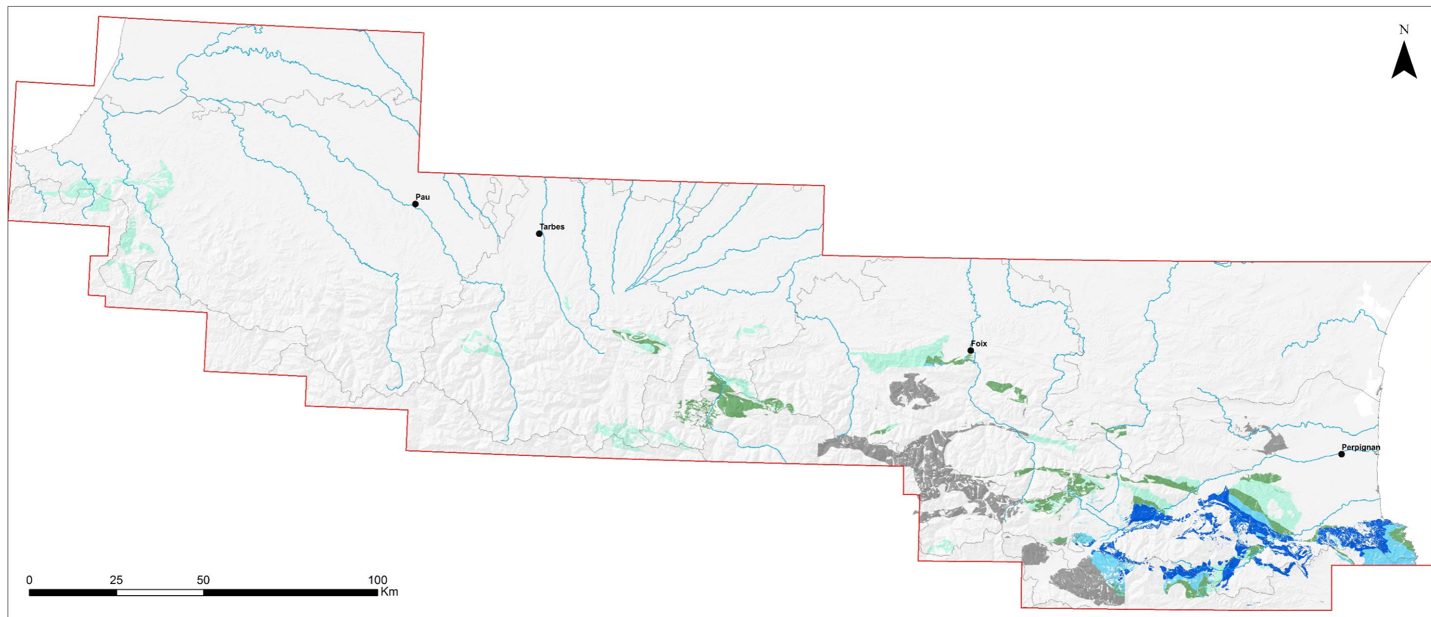
Carte géologique de l'évènement " Phase rhéique " (EG_8264) [Ordre 2] ammorçant la Divergence Varisque (EG_8775) [Ordre 2] . En vert : Bassin de la plateforme Nord Gondwaniennne des Formation d'Err et de Valcébollère ainsi que leur équivalent dans les Pyrénées Centrales du Groupe de Jujols; en turquoise : bassin marge passive épisode Rift to Drift équivalent à la Formation de Serdynia et les équivalent dans les Pyrénées Centrales et Occidentales ; (En bleu: le bassin extensif tardi-cadomien). Les zones en gris sont les roches du même âge dont l'origine du dépôt n'a pas pu être clairement identifiée par manque de données permettant de caractériser les événements à l'origine de ces dépôts.
