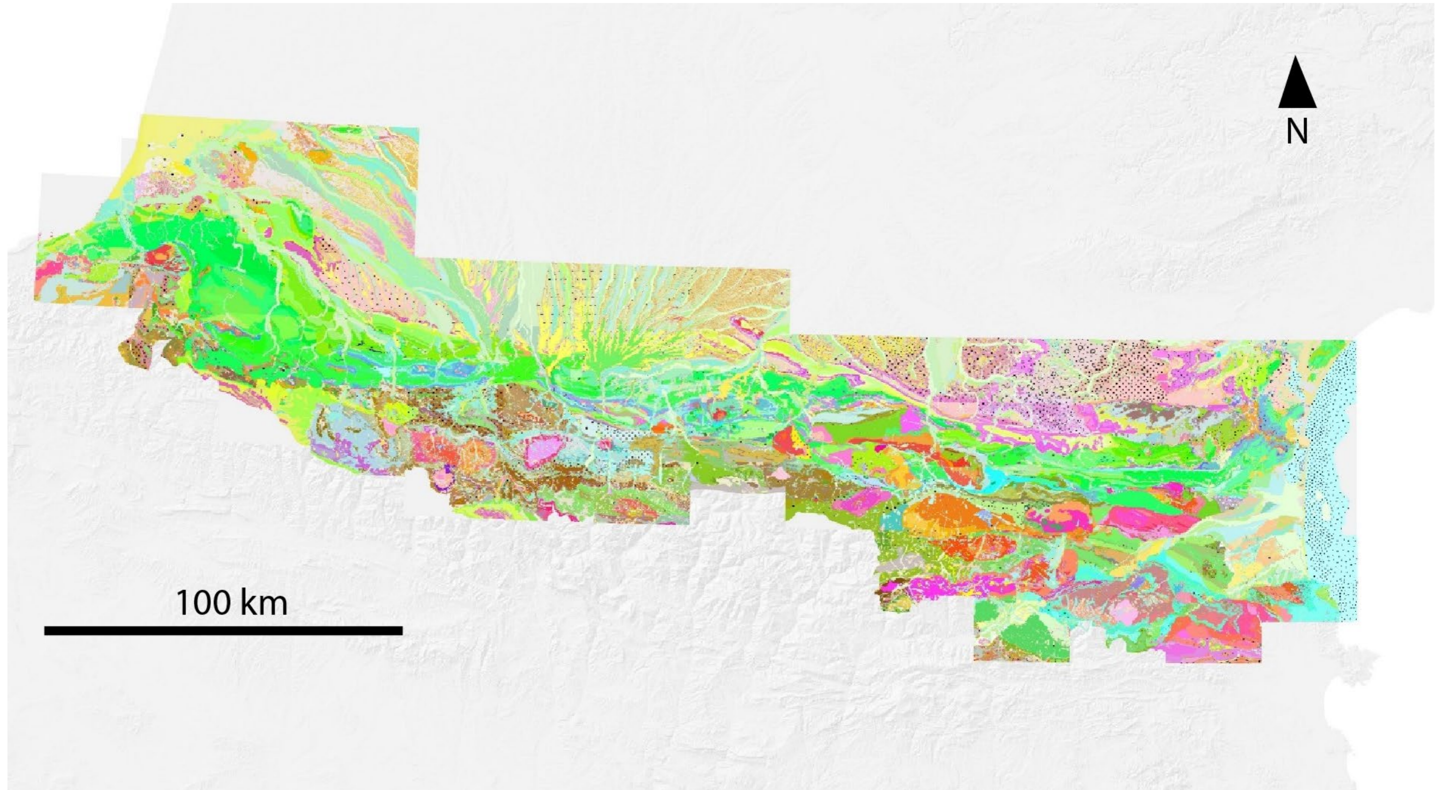
Carte simplifiée des formations géologiques de type "formation/membre" identifiées dans le cadre du chantier RGF-Pyrénées
