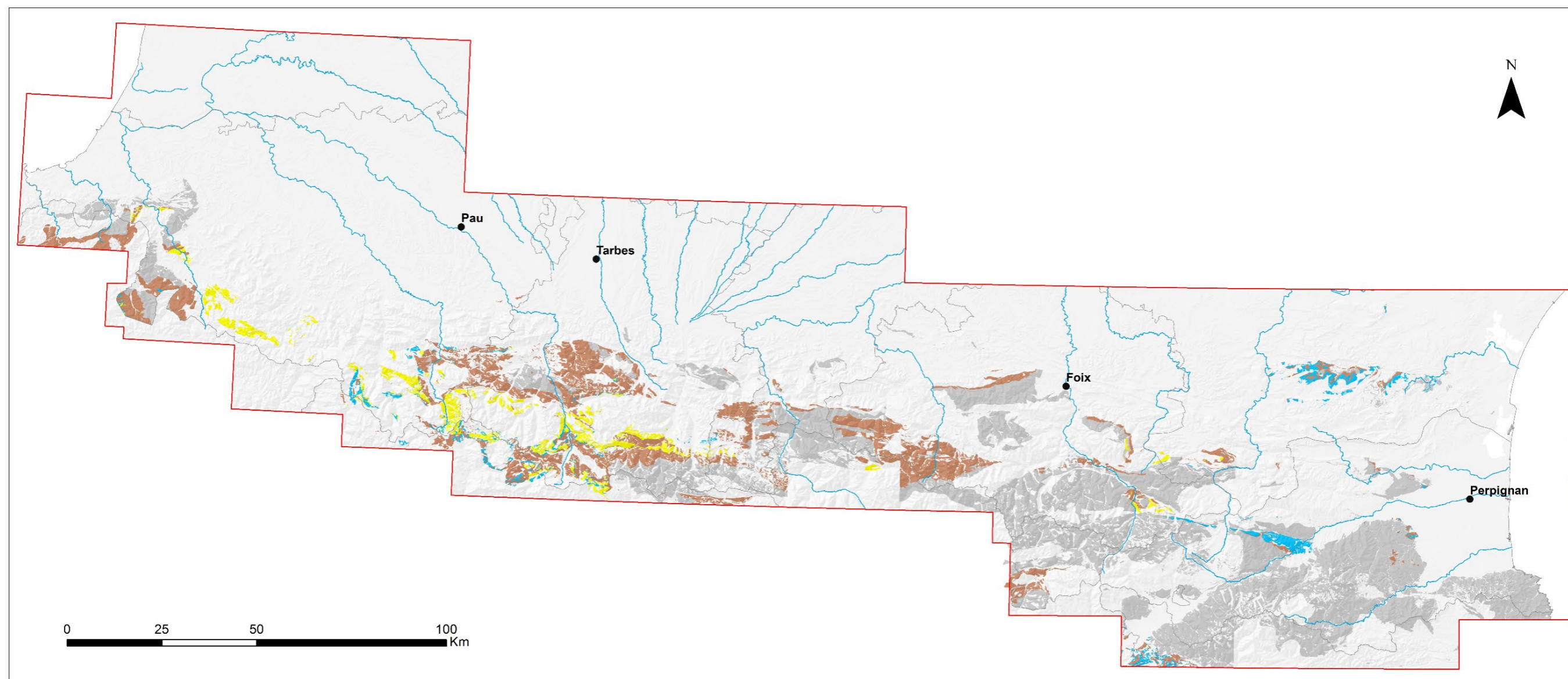
Carte géologique de l'évènement Bassin détritique intermédiaire du Dévonien (EG_8742) [Ordre 3] en jaune, soit les dépôts de la Formation Sia-Lariste ; et de l'évènement Bassin carbonaté intermédiaire du Dévonien (EG_8746) [Ordre 3] en bleu clair, soit les dépôts des Formations Larrue et Villefranche ou équivalents. L'ensemble de ces évènements sont intervenus au cours de la Convergence Varisque (EG_8269) [Ordre 1] et plus spécifiquement de l' Ouverture Paléotéthys (EG_8699) [Ordre 2] .
