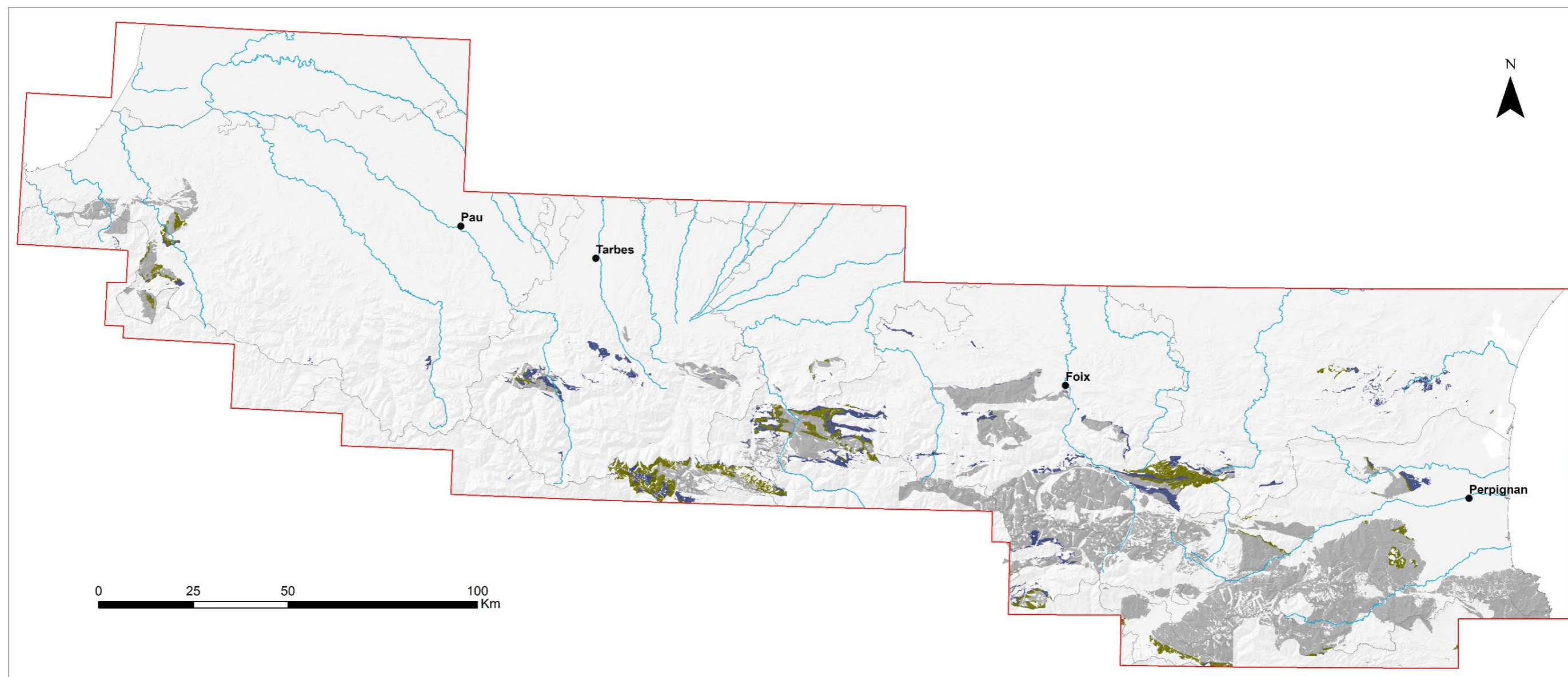
Carte géologique des événements “ Plateforme mixte de l’Ordovicien Supérieur (EG_8740) [Ordre 3] ” en verdâtre, soit les dépôts associés à la phase Sardes : et de l’évènement “ Rampe dysoxique du Silurien (EG_8776) [Ordre 3] ” en bleu marine, soit les dépôts associés au Climax de la Divergence Varisque (EG_8775) [Ordre 2] . Les zones en gris sont les roches dont les protolithes sont d’âge antérieur à ces événements.
