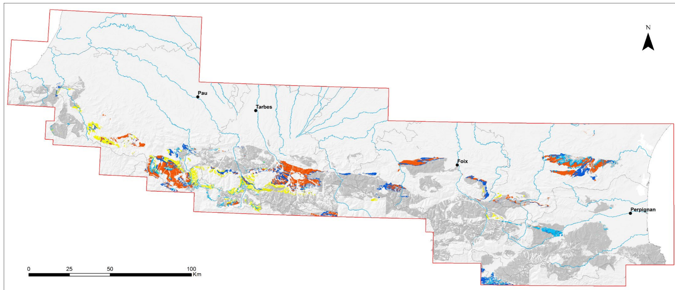
Carte géologique de l'évènement " Bassin syn-orogénique (faciès Culm) des Pyrénées (EG_8267) [Ordre 3] " en orange qui enregistre sous forme de dépôt la Phase Orogénique Varisque (EG_8268) [Ordre 2] . Les dépôts de ces bassins se mettent en place en contact avec les dépôts précédents appartenant aux évènements " Bassin détritico-intermédiaire du Dévonien (EG_8742) [Ordre 3] " en jaune, " Rampe carbonatée de la marge Paléotéthys (EG_8743) [Ordre 3] " en bleu clair et " Rampe carbonatée de la marge Paléotéthys (EG_8743) [Ordre 3] " en bleu foncé correspondant aux Calcaires Griottes et Lydiennes.
