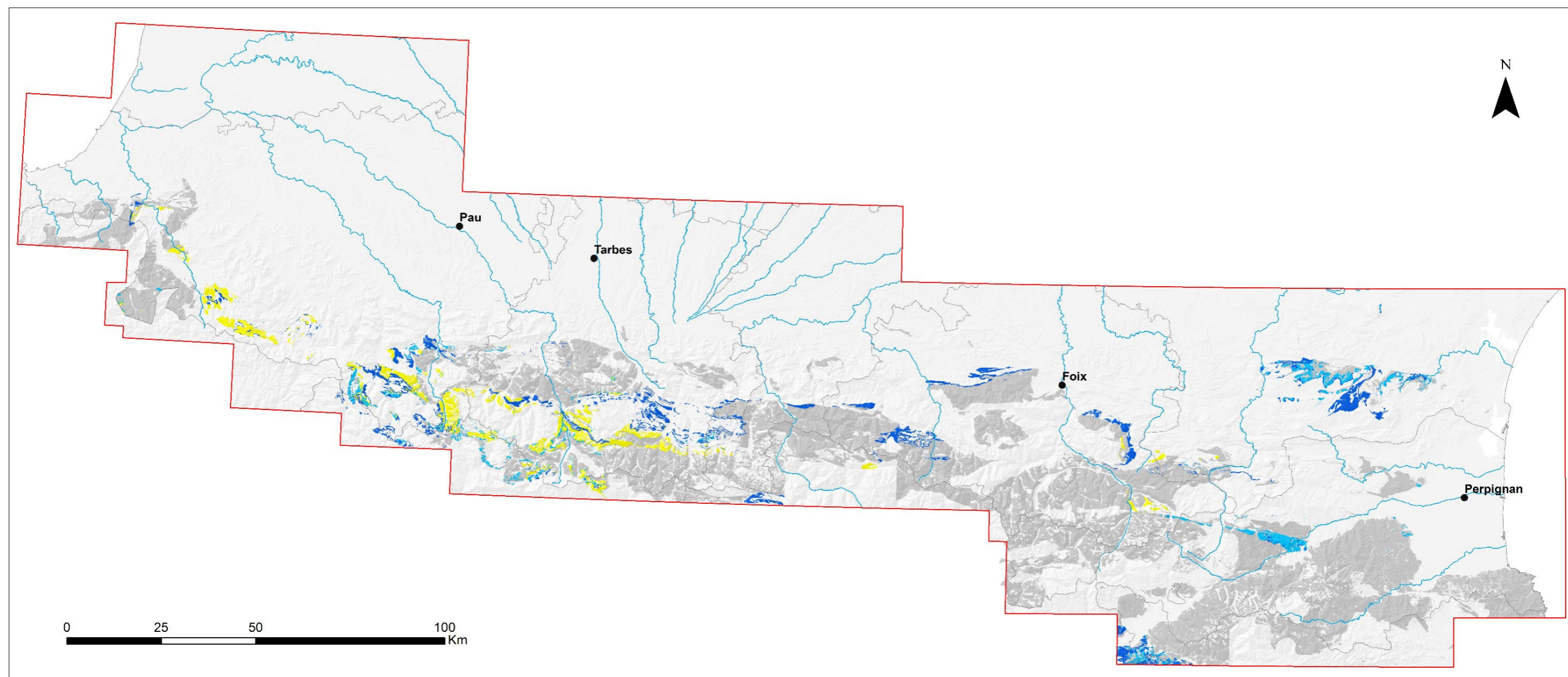
Carte géologique de l'évènement "Bassin détritique intermédiaire du Dévonien (EG_8742) [Ordre 3]" en jaune, de l'évènement Bassin carbonaté intermédiaire du Dévonien (EG_8746) [Ordre 3] en bleu clair, et finalement de l'évènement "Rampe carbonatée de la marge Paléotéthys (EG_8743) [Ordre 3]" en bleu foncé correspondant aux Calcaires Griottes et Lydiennes qui terminent l'Ouverture Paléotéthys (EG_8699) [Ordre 2].
