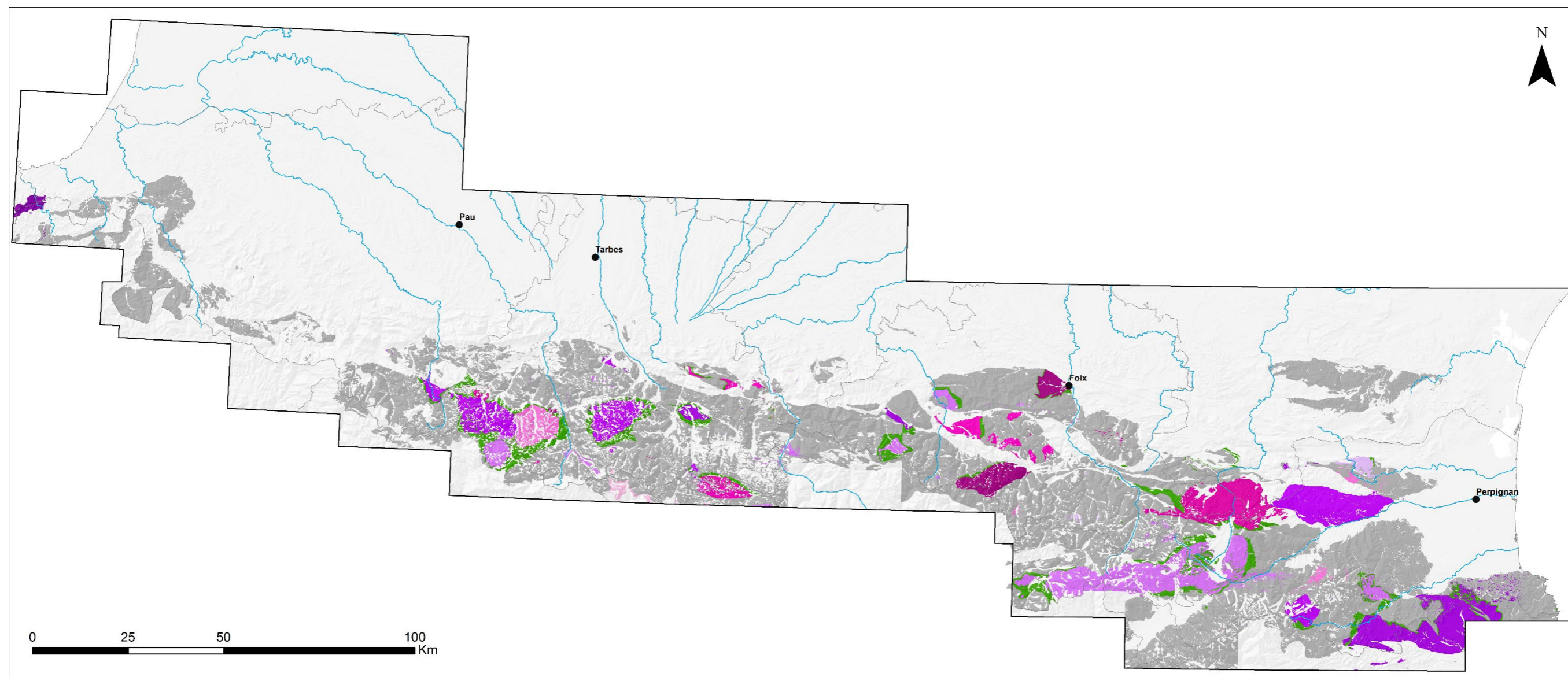
Carte géologique de l'évènement « Magmatisme Tardi-Varisque (EG_8195) [ordre 3] ». Dans les différentes gammes de roses-violets, il s'agit des différents complexes plutoniques (ex : Querigut, Mont-Louis, Caunterets, Néouvielle, Bordères-Louron, etc.) ; en vert : auréoles de métamorphisme de contact qui sont individualisées pour chacun des différents complexes, et rattaché à cet évènement magmatique. Cette carte montre que des évènements métamorphiques et plutoniques (Ordre 4) peuvent être réunis au sein d'un évènement magmatique (Ordre 3) qui lui-même est rattaché à un évènement géodynamique « Phase Tardi-Varisque (Ordre 2) » appartenant au stade de convergence Varisque (Ordre1). Les zones en gris sont les roches dont les protolithes sont d'âge antérieur à cet évènement de magmatisme.
