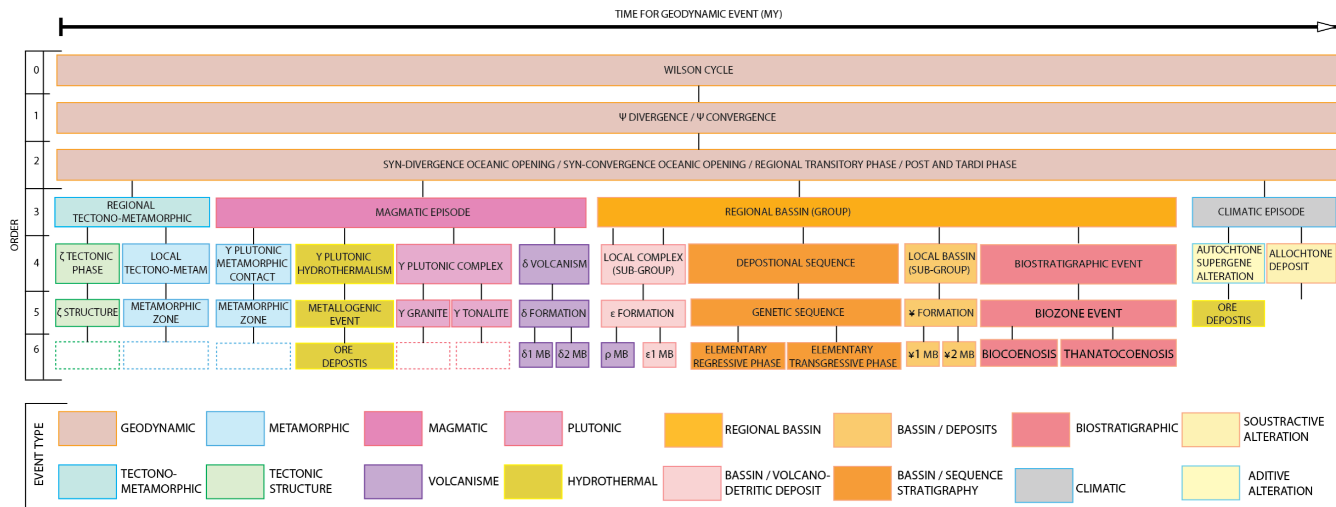
Figure 18 : Vue simplifiée des types d'évènements géologiques à différents ordres et de leur hiérarchie.
