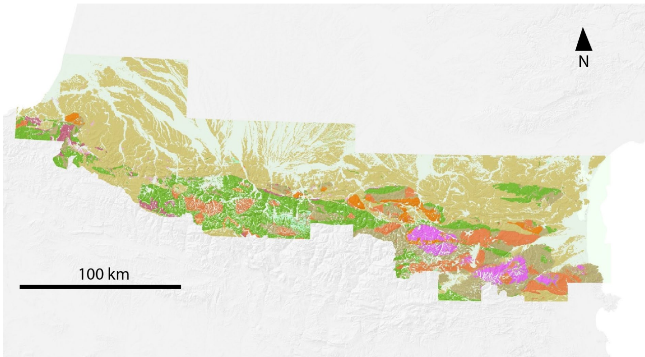
Figure 6 : Carte simplifiée des unités lithostratigraphiques de type "supergroupes" identifiées dans le cadre du chantier RGF-Pyrénées
