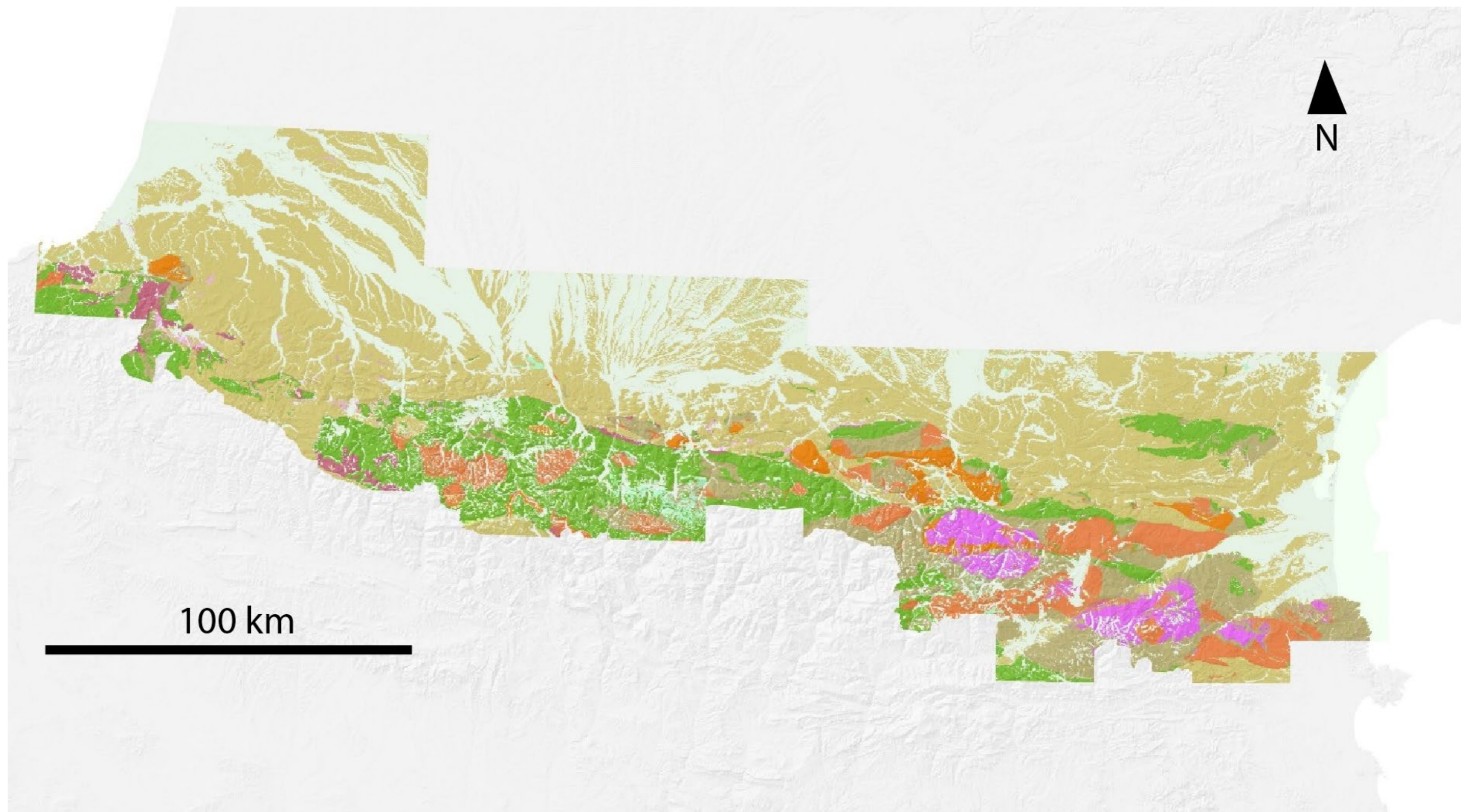
Carte simplifiée des formations géologiques de type “super-groupes” identifiées dans le cadre du chantier RGF-Pyrénées
