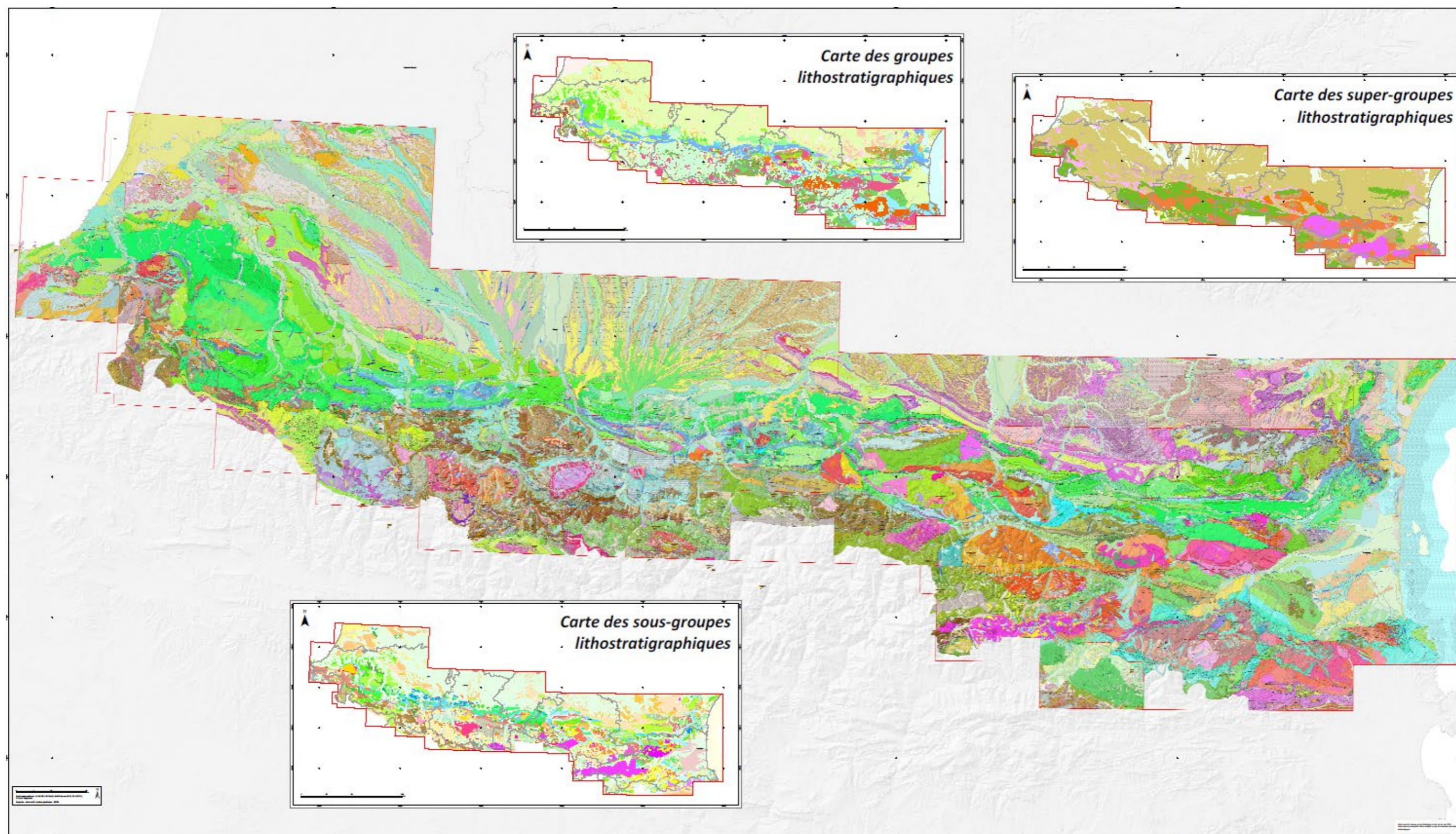
Carte géologique RGF chantier Pyrénées.
