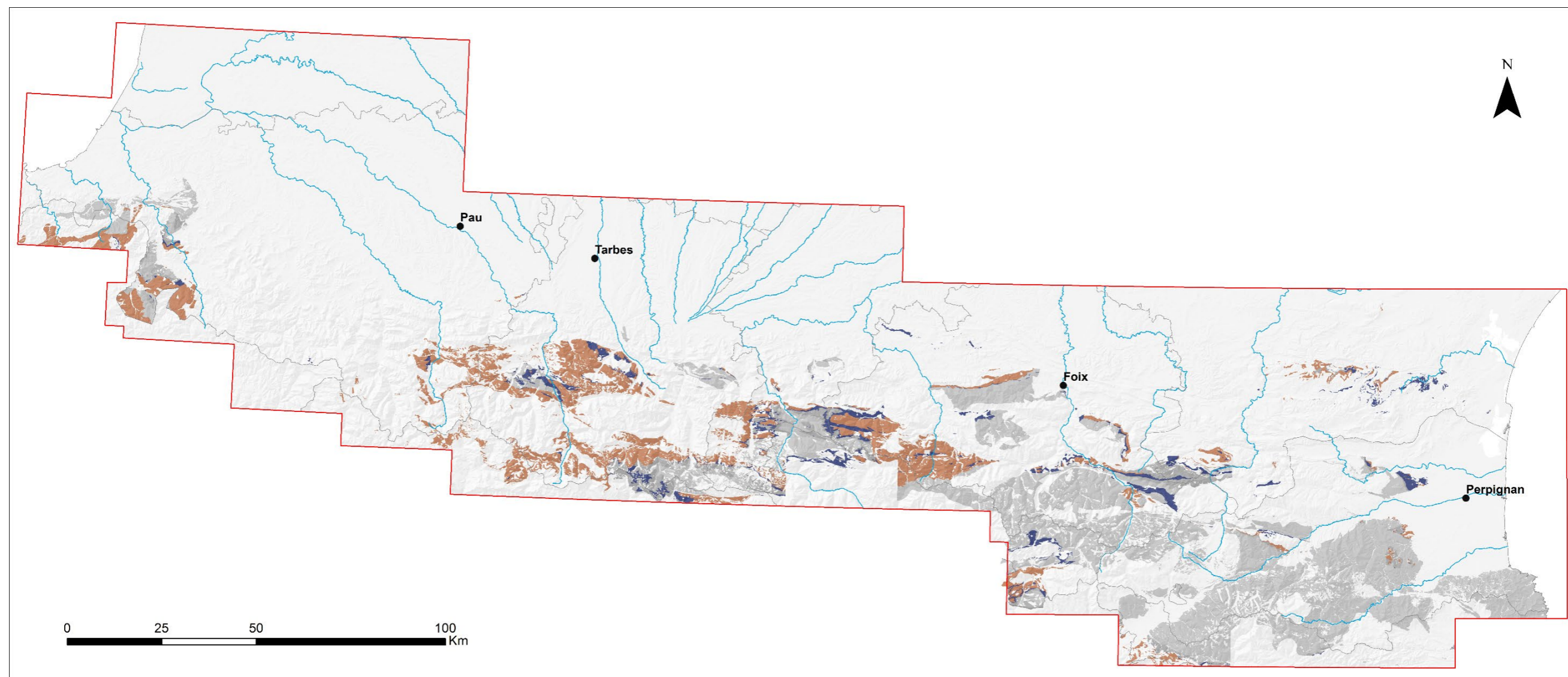
Carte géologique de l'évènement "Groupe inférieur-moyen du Dévonien (EG_8741) [Ordre 3]" et de l'évènement "Groupe des faciès de transition du Siluro-Dévonien (EG_8745) [Ordre 3]" associés au début de la Convergence Varisque (EG_8269) [Ordre 1] et plus spécifiquement de l'Ouverture Paléotéthys (EG_8699) [Ordre 2].
