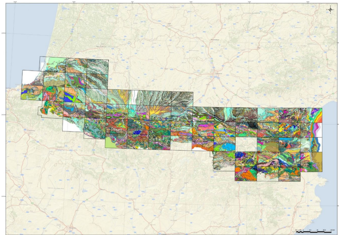
Figure 4. Cartes 1/50 000 du chantier RGF Pyrénées : 58 coupures à 1/50 000 vectorisées et une manquante en 2014, la feuille d'Ax-Les-Thermes. Cette dernière coupure a été réalisé au cours du chantier et la maquette a été présentée en 2019 lors du colloque final de restitution du chantier RGF.
