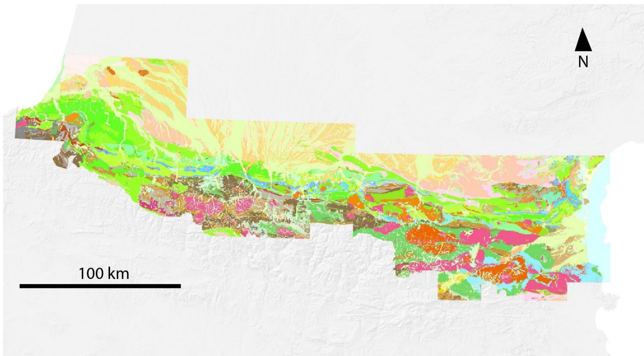
Figure 7 : Carte simplifiée des unités lithostratigraphiques de type "groupes" identifiées dans le cadre du chantier RGF-Pyrénées
