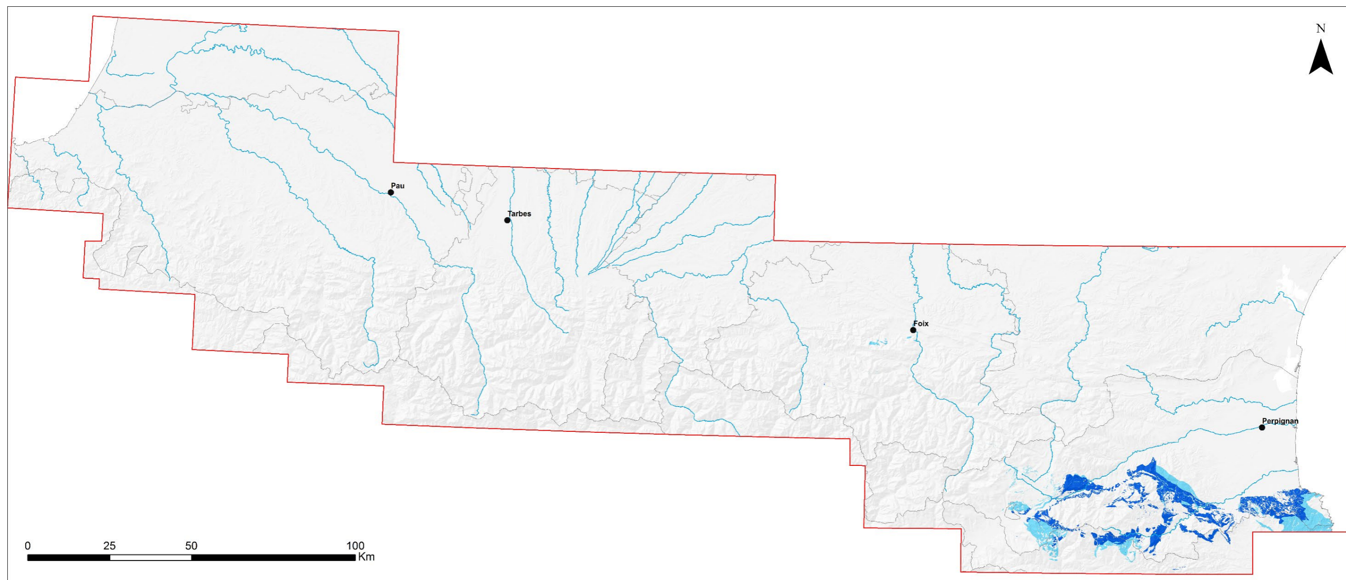
Carte géologique de l'évènement " Bassin extensif tardi-cadomien " (EG_8604) [Ordre 3]. En bleu foncé, les dépôts du sous-groupe de Nùria; et en bleu clair, les dépôts du sous-groupe de Setcasas.
