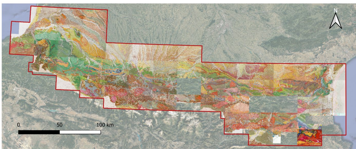
Figure 1 : Emprise du chantier RGF Pyrénées : 59 coupures à 1/50 000 dont 2 feuilles encore non validées par le CCGF (St Paul de Fenouillet, et Aspet) et une carte manquante (Ax-Les-Thermes). Cette dernière coupure a été réalisée au cours du chantier et la maquette a été présentée en 2019 lors du colloque final de restitution du chantier RGF.
