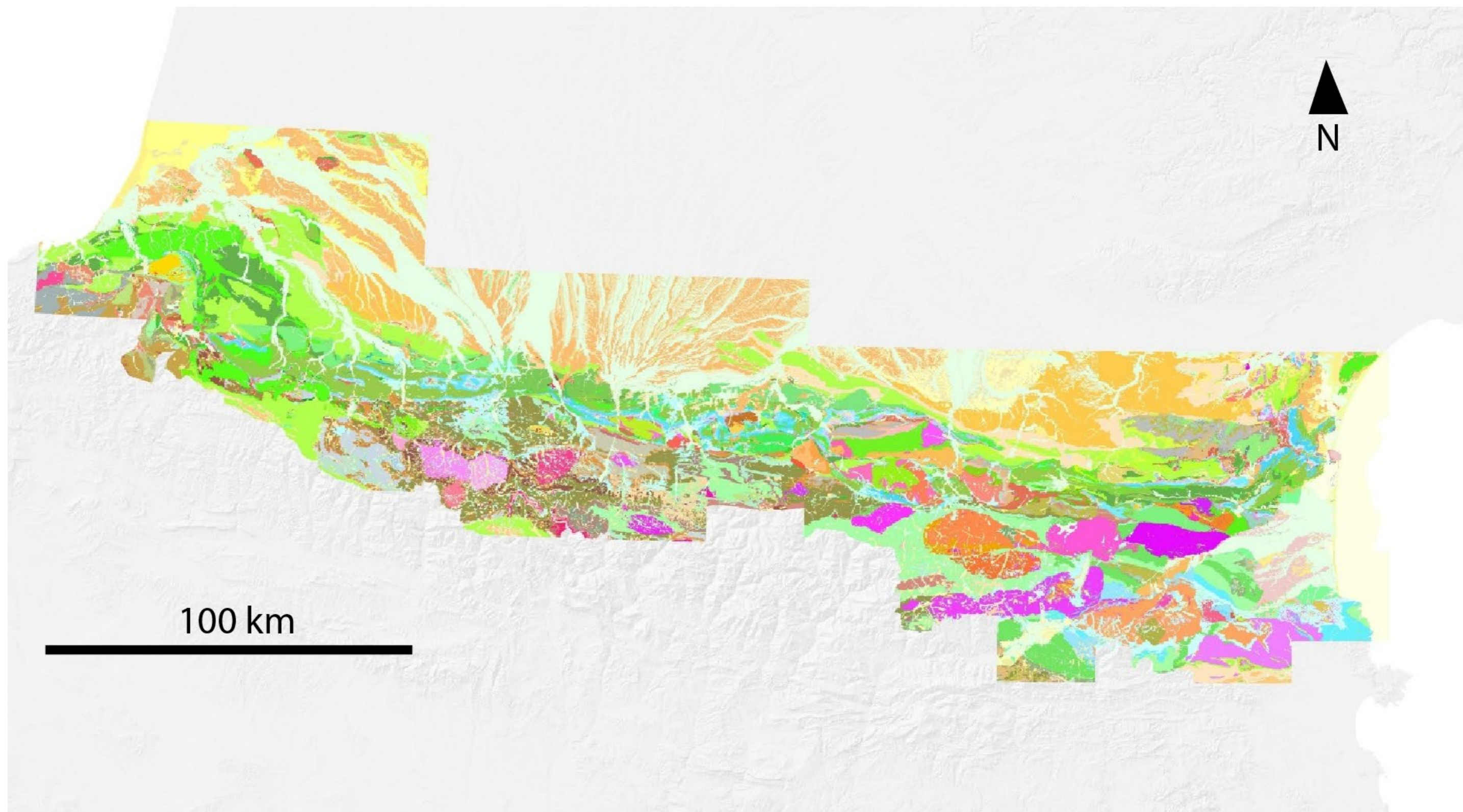
Carte simplifiée des formations géologiques de type "sous-groupes" identifiées dans le cadre du chantier RGF-Pyrénées
