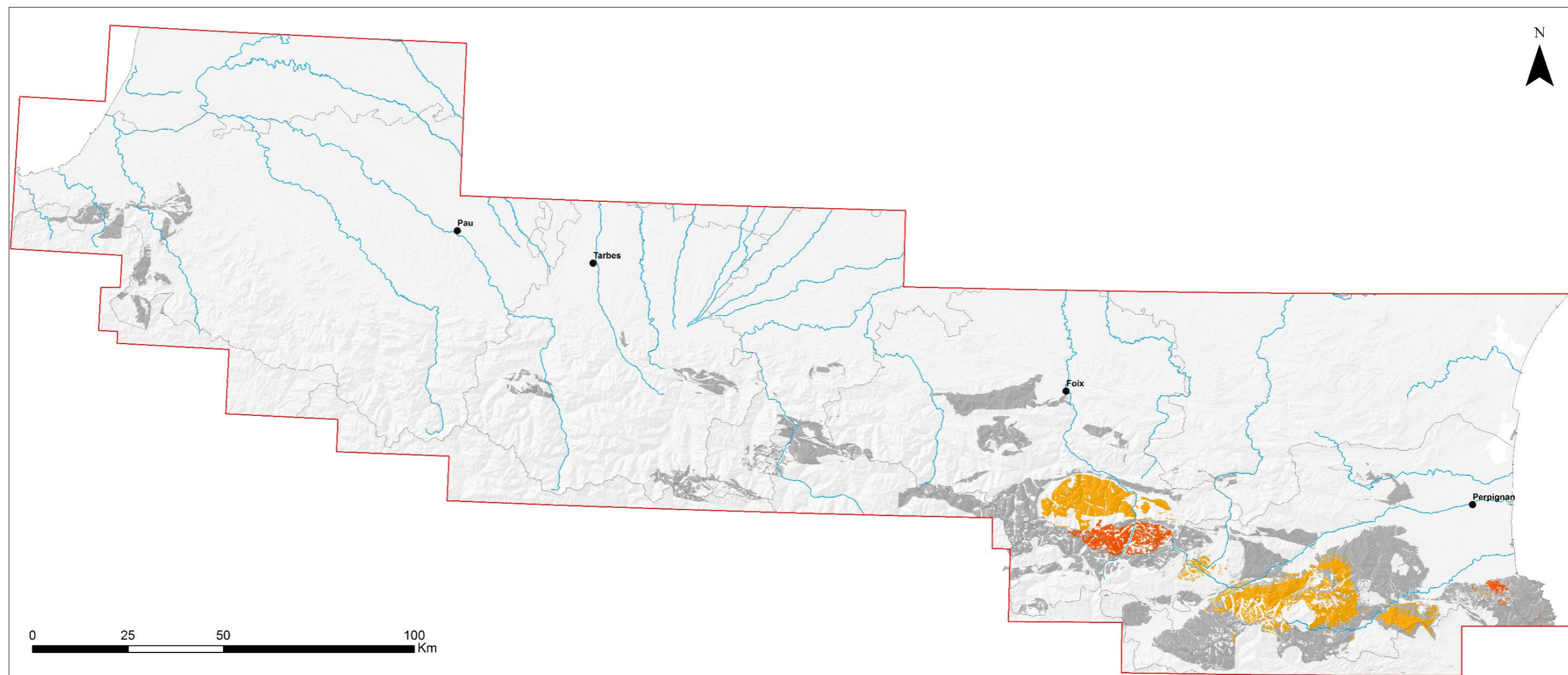
Carte géologique de l'évènement « Plutonisme Sarde (EG_8197) [ordre 3] ». Dans les différentes gammes d'orange, il s'agit des différents complexes plutoniques ordovicien (Aston, Hospitalet, Canigou-Roc de Frausa, Albères). Les zones en gris sont les roches dont les protolithes sont d'âge antérieur à cet évènement de magmatisme.
