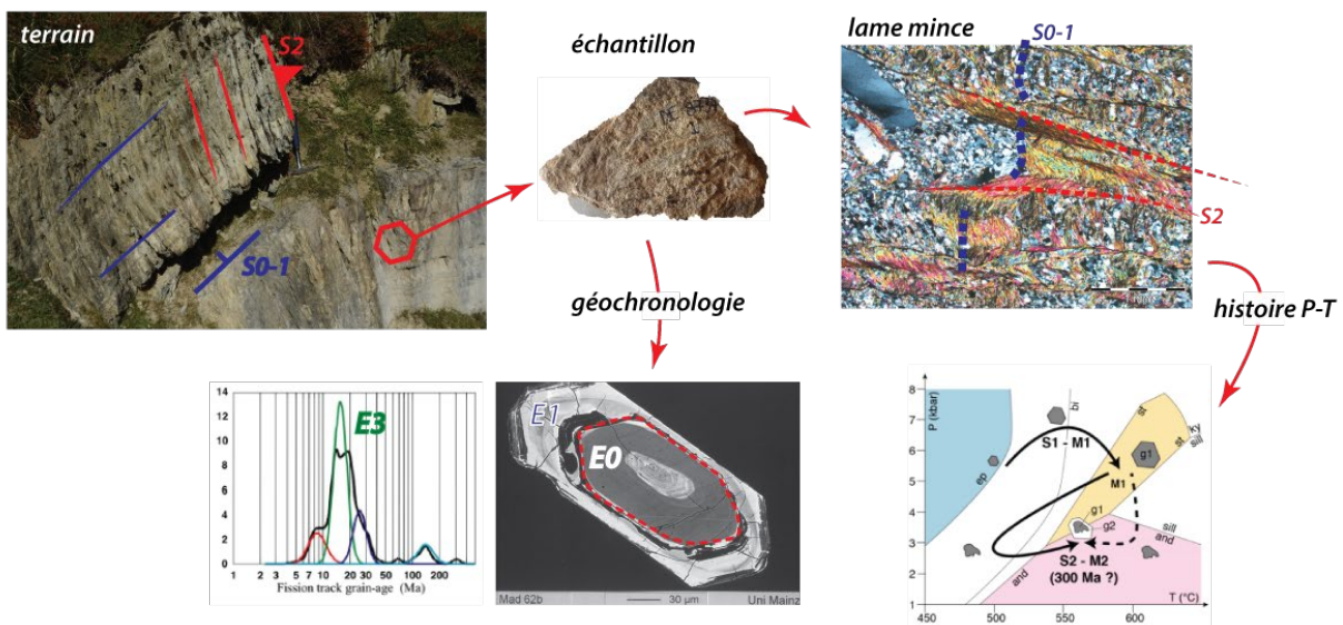
Figure 19 : L'évènement géologique est le liant de toutes les informations géologiques. Les données sont « factuelles », les évènements sont interprétatifs. Un ou plusieurs évènements géologiques peuvent être observés sur un échantillon ou un affleurement. Ces évènements peuvent être représentés par des mesures (mesures structurales), des analyses (pétrologiques, géochimiques, géochronologiques).
